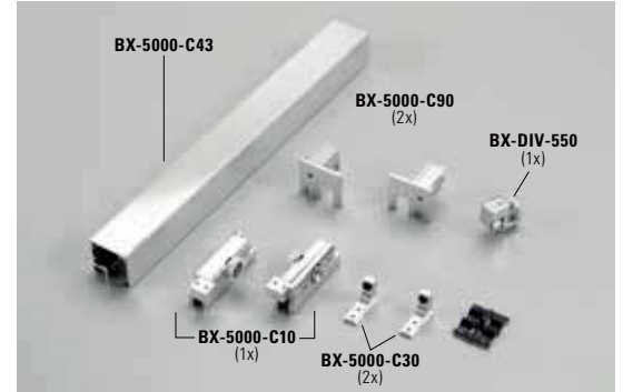
CARATTERISTICHE COMPONENTI FEATURES COMPONENTS - EIGENSCHAFTEN EINZELTEILE
