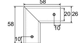
B-173 €► BX.336 • Raccordo regolabile per tubo Ø 19 mm. • Adjustable connector for Ø 19 mm tube. • Verbinder für 19 mm Rohr Verstellbar. CR - NS
