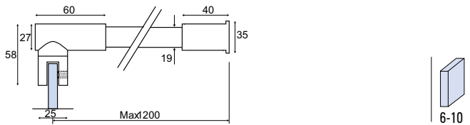
B-167 €► BX.331 • Fermavetro snodata a muro. • Ends Forged brass. • Halterungen für Stabilisationsstange. CR - NS
