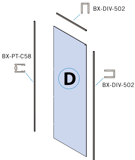
BX-DIV-ANT-D ANTA FISSA LATERALE D FLATERAL FIXED PANEL D SEITENTEIL D
