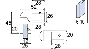
B-165 €► BX.334 • Raccordo a 90° per tubo Ø19 mm. • 90° connector for 19 mm tube. • Rohrverbinder 90° für Rohr Ø 19 mm. CR - NS
