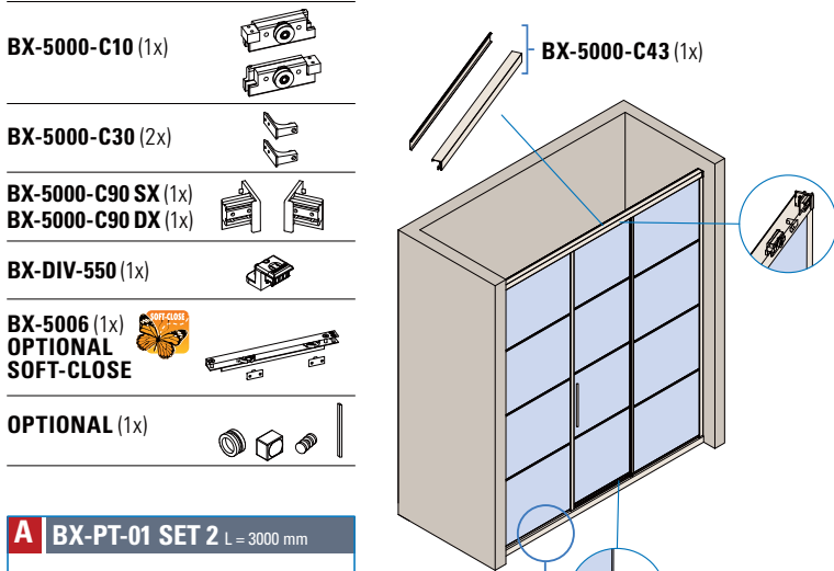
CARATTERISTICHE COMPONENTI FEATURES COMPONENTS - EIGENSCHAFTEN EINZELTEILE
